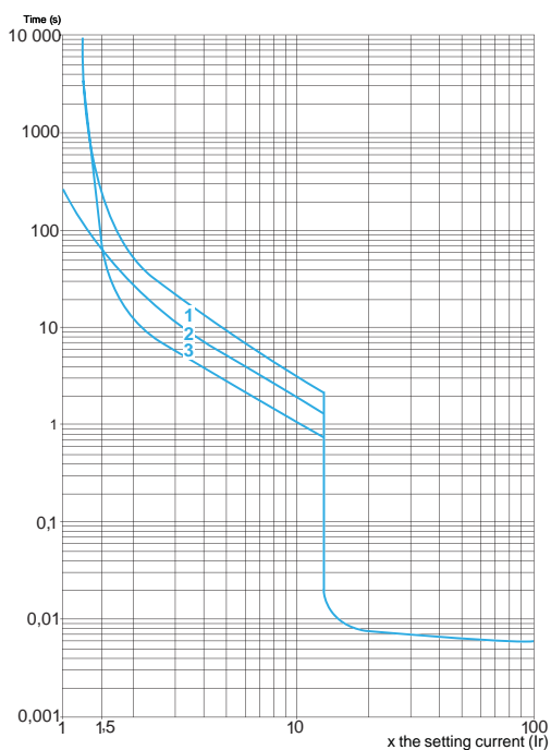
Kioldási jelleggörbe
