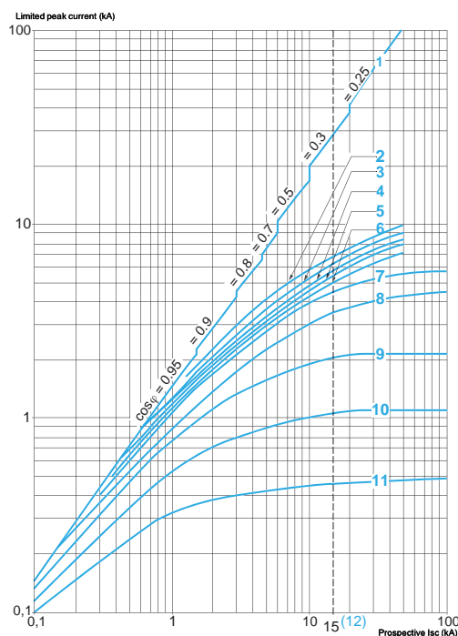
Áramkorlátozási jelleggörbe
